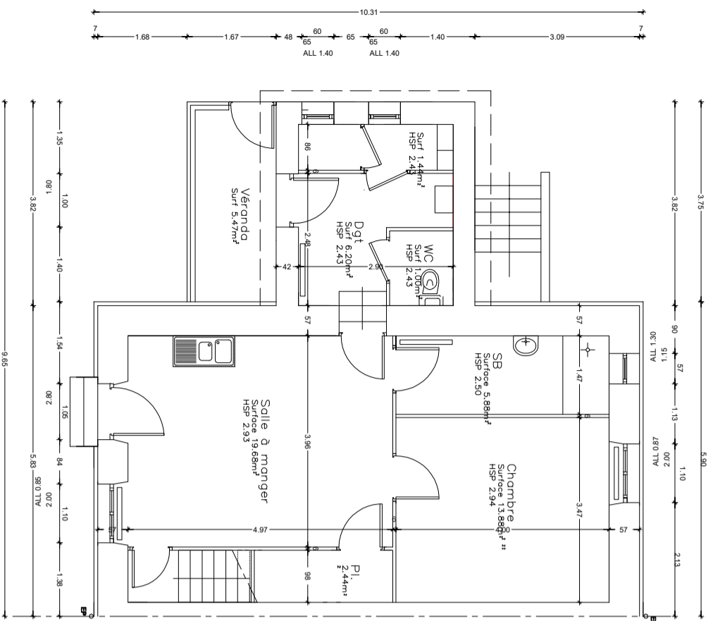
RDC
